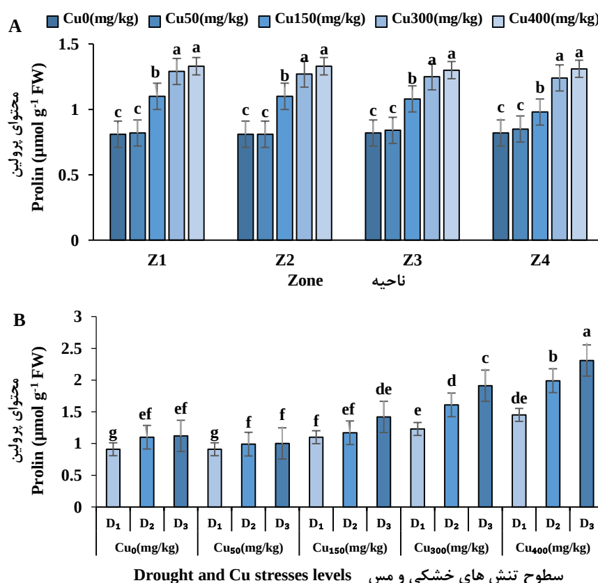
شکل ۵. میانگین اثرات متقابل تنش مس و منطقه بر محتوای پرولین در F. parviflora (A). میانگین اثرات متقابل مس و تنش خشکی بر محتوای پرولین در F. parviflora (B). D1: شاهد، D2: ۵۰٪ ظرفیت زراعی، D3: ۲۵٪ ظرفیت زراعی. Z1: ناحیه ۱ با غلظت ۵۰ میلی گرم مس بر کیلوگرم، Z2: ناحیه ۲ با غلظت ۱۵۰ میلی گرم مس بر کیلوگرم، Z3: ناحیه ۳ با غلظت ۳۰۰ میلی گرم مس بر کیلوگرم و Z4: ناحیه ۴ با غلظت ۴۰۰ میلی گرم مس بر کیلوگرم. گروه‌های واجد حروف یکسان، با توجه به آزمون دانکن، تفاوت معنی‌دار ( P \leq 0.01 ) ندارند.
